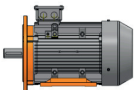
IMB35
